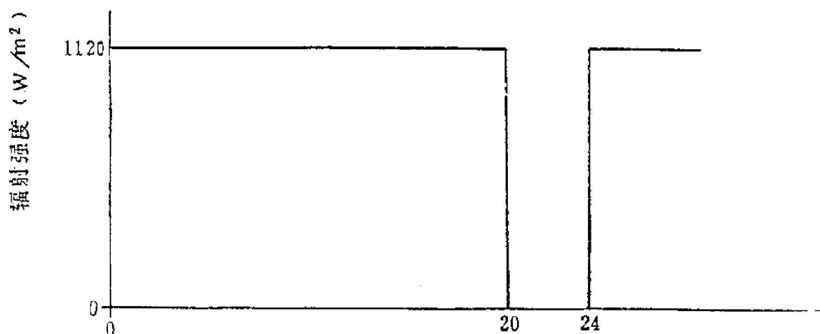
图2 稳态长期光化学效应日循环
