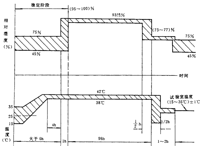
图 2 恒湿试验图
