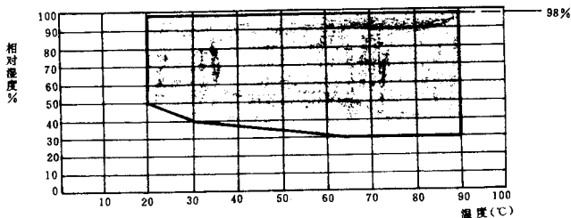
图 1 湿度范围图
