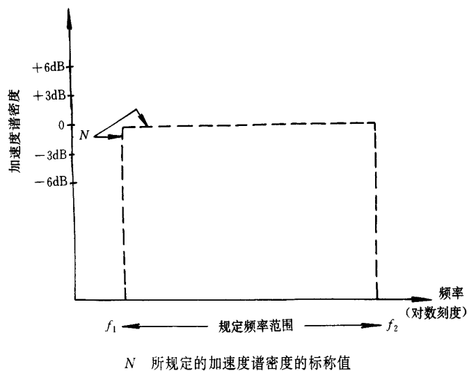
图 2 加速度谱密度的频谱
